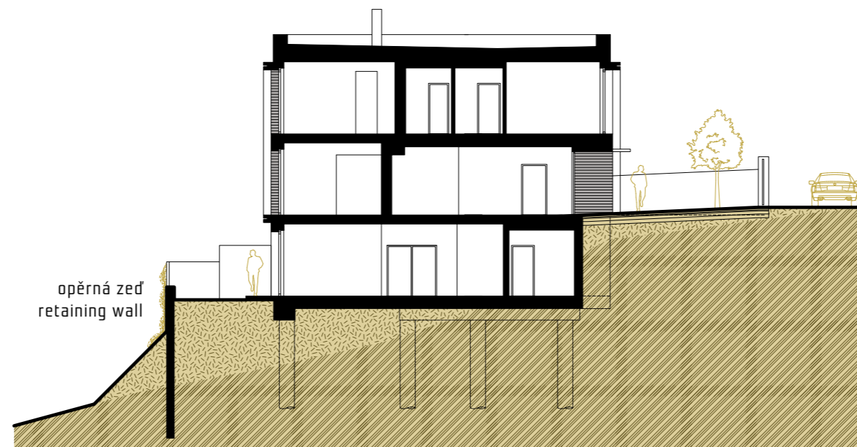
podélný řez | section view
