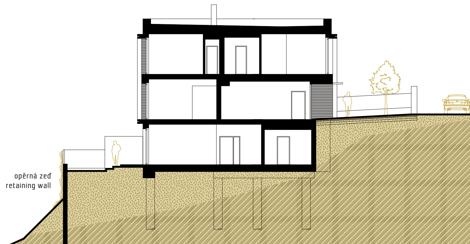
podélný řez | section view
